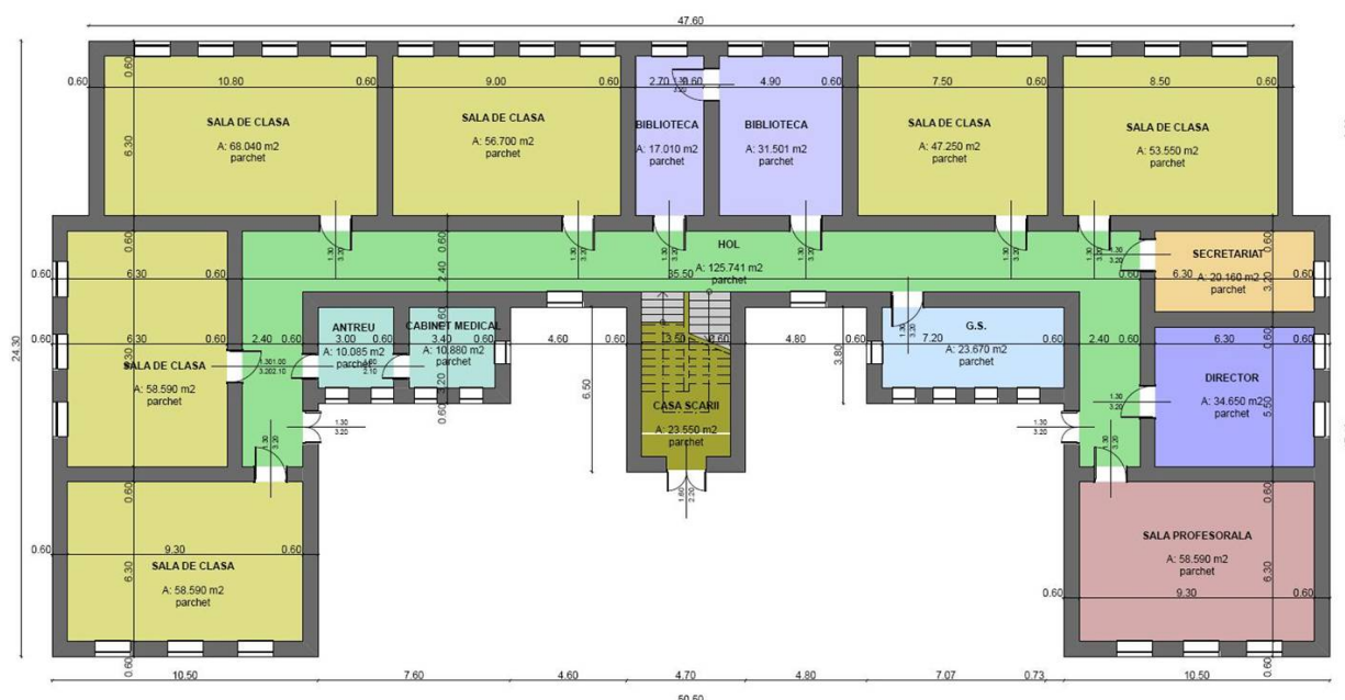
Fig. 93 Planul școlii - parter
