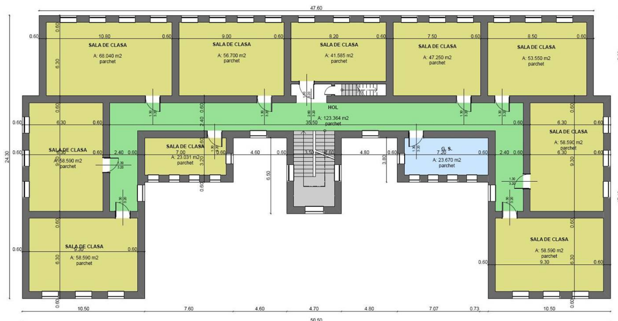
Fig. 94 Planul școlii - etaj
